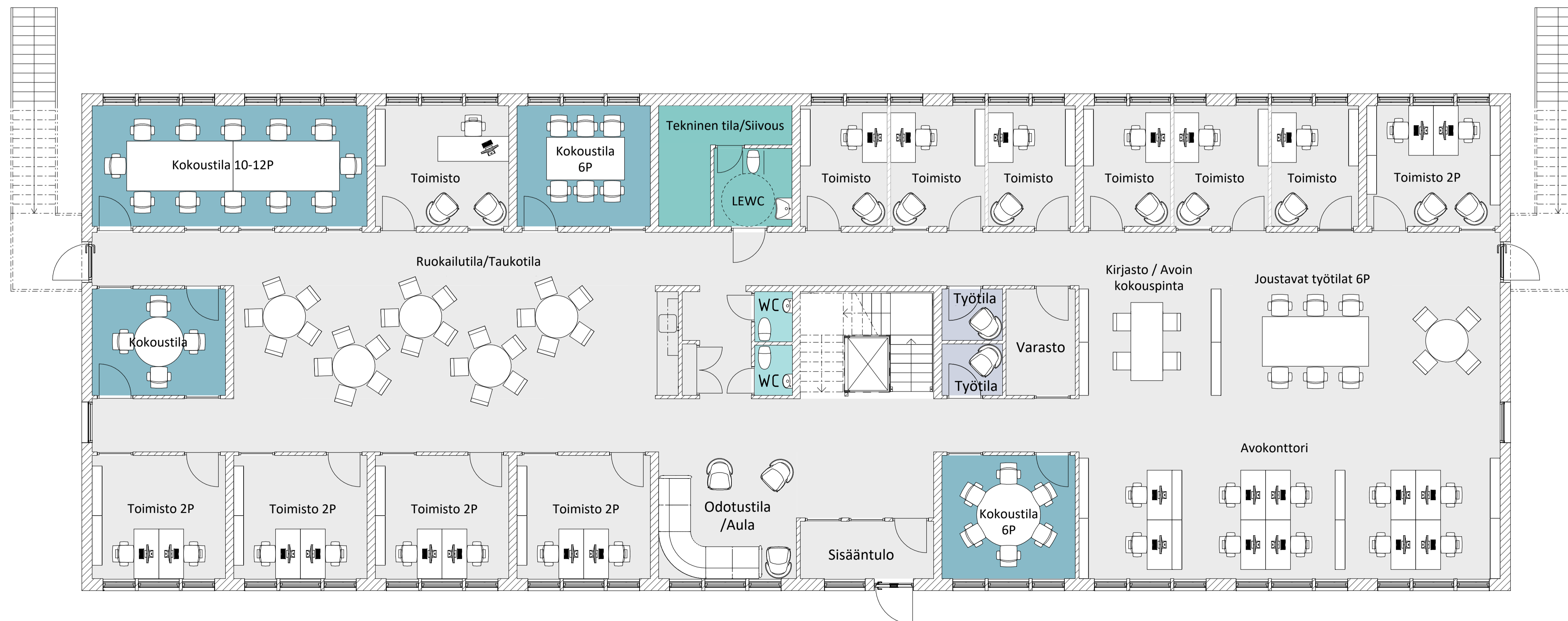
1. KERROS
